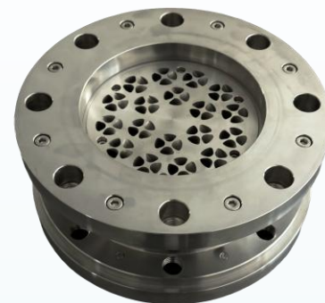
FB-M150A-SUS316L (JIS10K 150Aフランジ)
