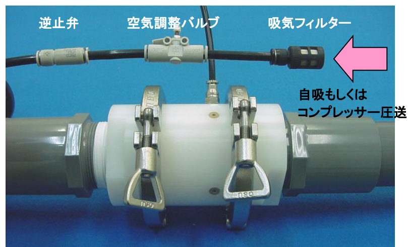
ファインバブル発生器 FB-M40A/M50A
