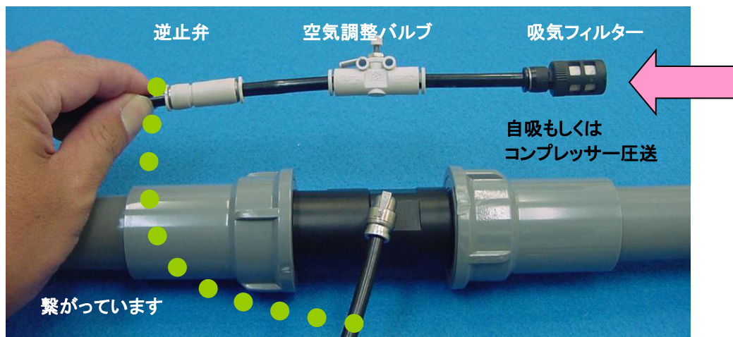
ファインバブル発生器 FB-S25AI
